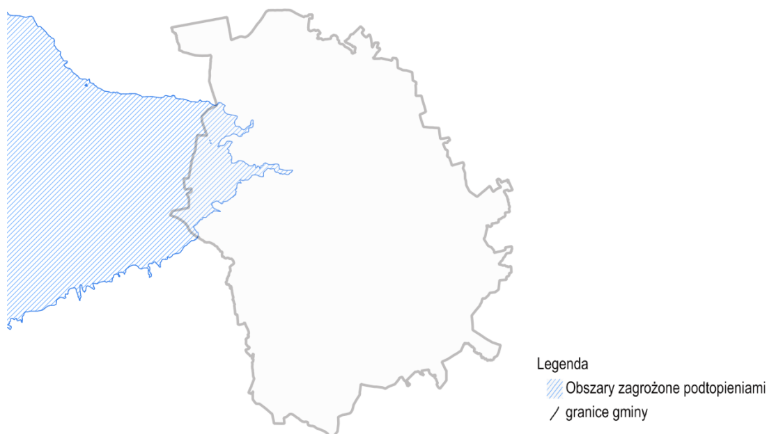
Rysunek 30. Obszar zagrożone podtopieniami na terenie gminy Pasłęk.
