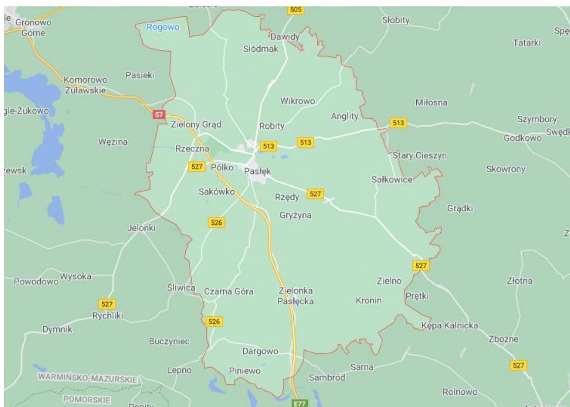
Rysunek 13. Układ głównych dróg na terenie Gminy Pasłęk.
