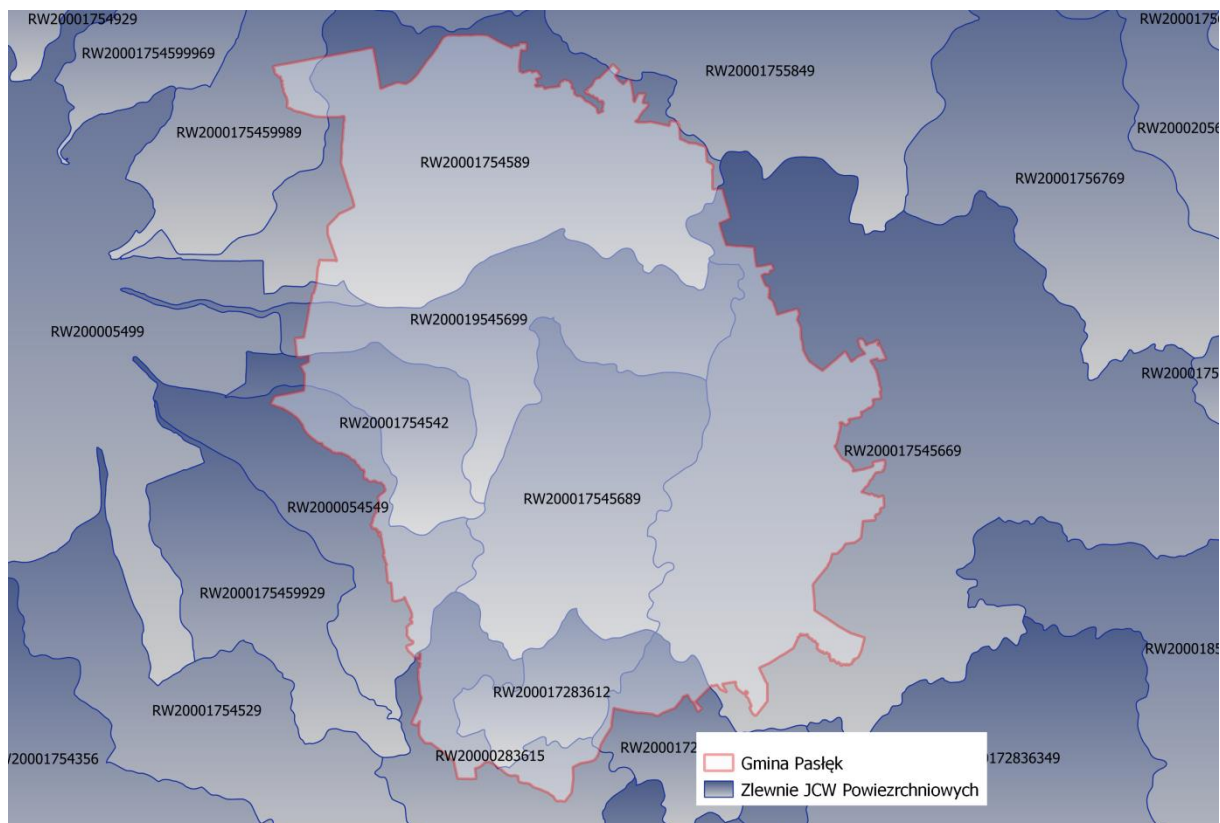
Rysunek 26. Zlewnie jednolitych części wód powierzchniowych na terenie Gminy Pasłęk. źródło: Geoportal, opracowanie własne
