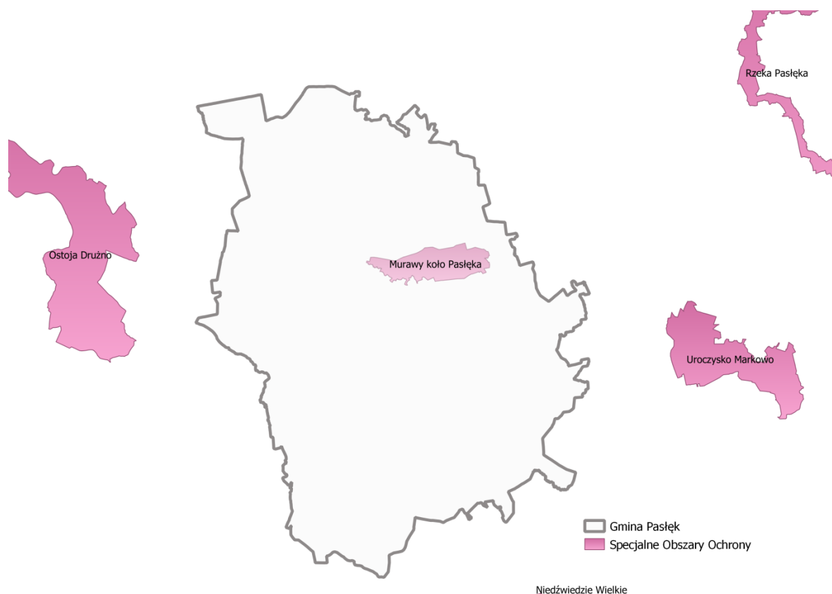
Rysunek 35. Obszar Natura 2000 „Murawy koło Pasłęka” źródło: Geoserwis; opracowanie własne
